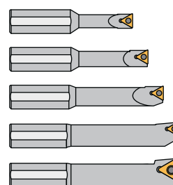
Tools for boring heads Werkzeuge für Bohrköpfe
